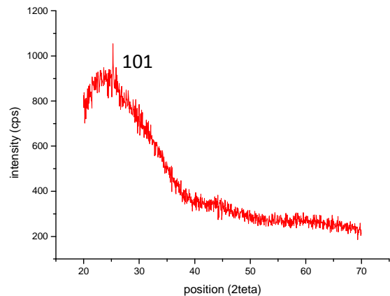
Fig.12: Diagramme de diffraction des rayons X (2θ variant entre 20° et 70°) de la couche mince de TiO 2 recuit à 500 °C pendant 1h.
