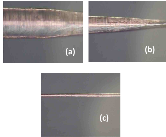
Fig. 4: Images (a), (b) et (c), obtenues par microscopie optique, représentent les variations du diamètre de la fibre optique après l'attaque chimique,
