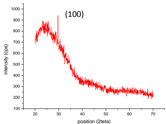
Fig.13 : Diagramme de diffraction des rayons X (2θ variant entre 20° et 70°) de la couche mince de ZnO recuit à 500 °C pendant 1h.
