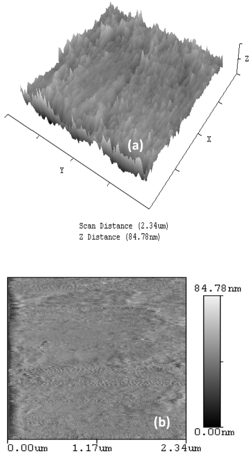
Fig.11: Images AFM de 10 couches minces de SiO 2 recuites pendant 1h à 450°C. (a) vue 3D et (b) vue 2D donnant la surface scannée
